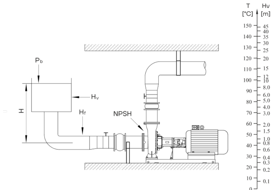
Рис. 7 Система с насосом
