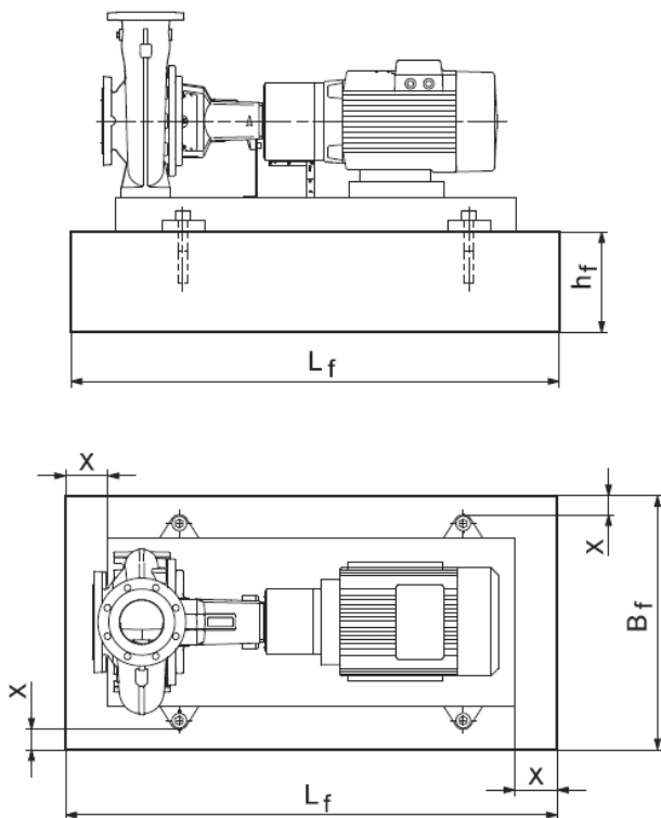
Рис.8 Фундамент.
