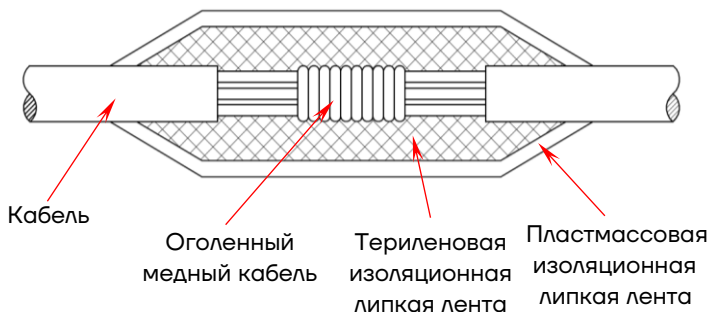
Рис. 9. Изоляция электрокабеля
