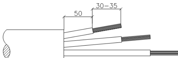
Рис. 7. Оголение электрокабеля
