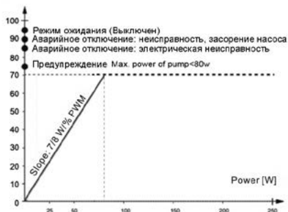
Рис 8. Логика сигнала обратной связи ШИМ
