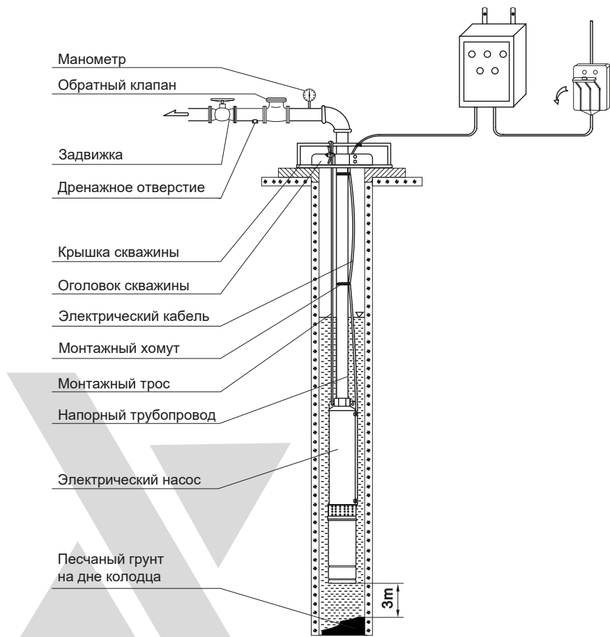
Схема установки
